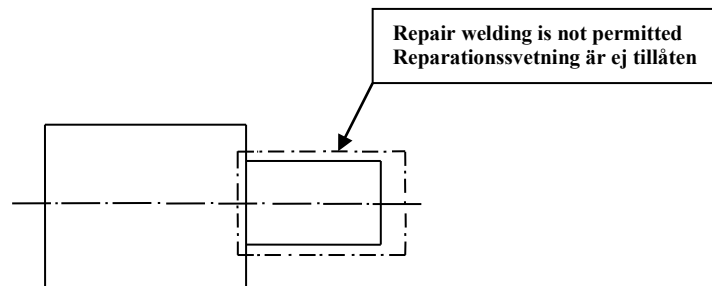
Ex. 5 Zone-marking of surfaces where the repair welding is not permitted Zonmarkering av ytor där reparationssvetsning ej är tillåten
